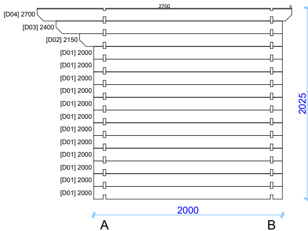
Wall D 1:40
