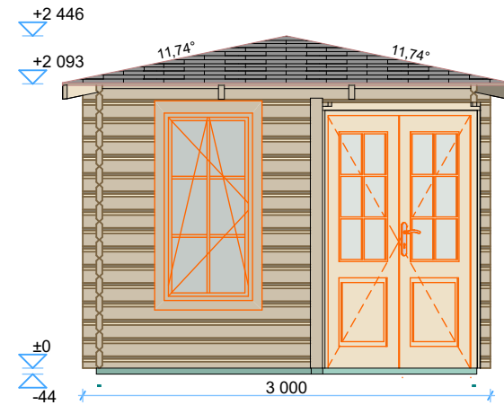
Right Elevation
